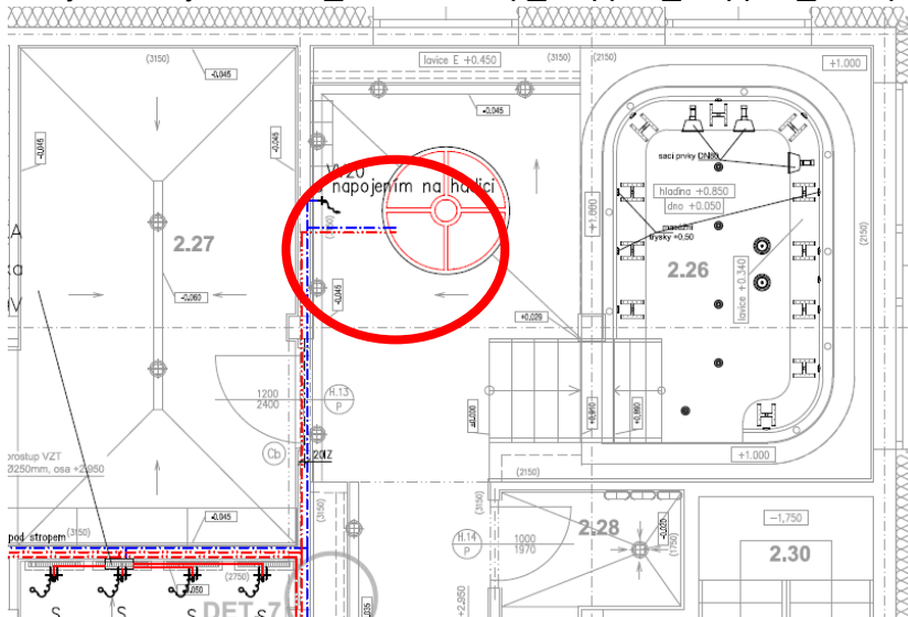
Nový stav, výkres 003_vodovod 2np_cropped_cropped_rev1.pdf:
