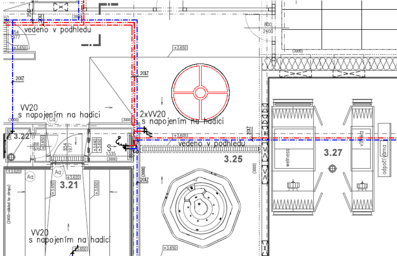
Původní stav, výkres 004_vodovod 3np_cropped_cropped.pdf
